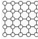
Figure 1: Система соседства — прямоугольная решетка
