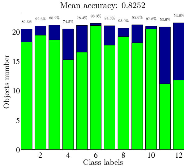
Рис. 3: Ручное выделение признаков.
