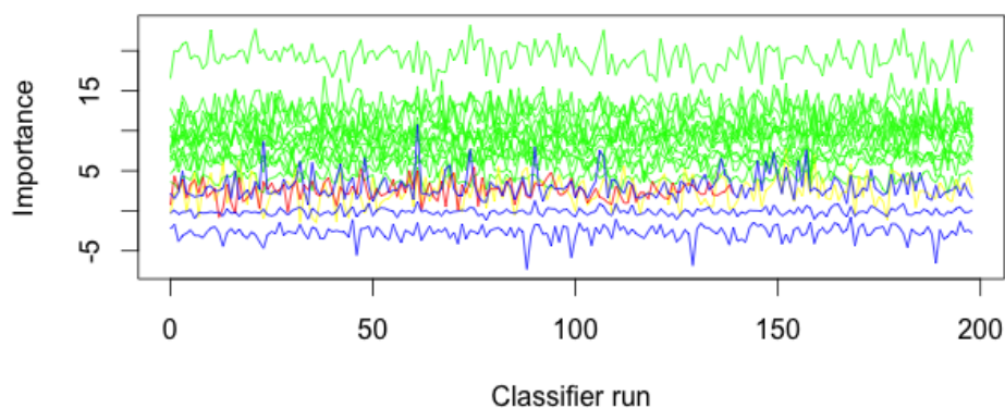
Рис. 5: важность признаков с помощью Boruta
